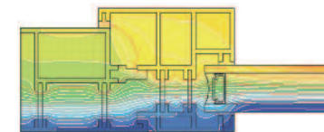
Schéma isothermique de l'intercalaire Warm Edge
