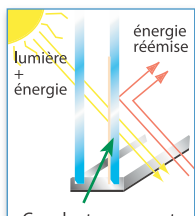
Couche transparente faiblement émissive
