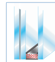
44.2/16/4 (reconnu par les assurances) (coef Ug=2,8) (Rw 33 db)
