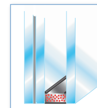
SP 10/16/4 (reconnu par les assurances) (coef Ug=2,8) (Rw 34 db)
