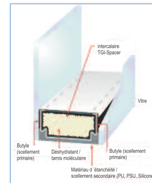
Coupe de l'intercalaire Warm Edge
