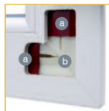
Insert soudé (a) solidaire des renforts métalliques (b) assurant la continuité du renforcement
