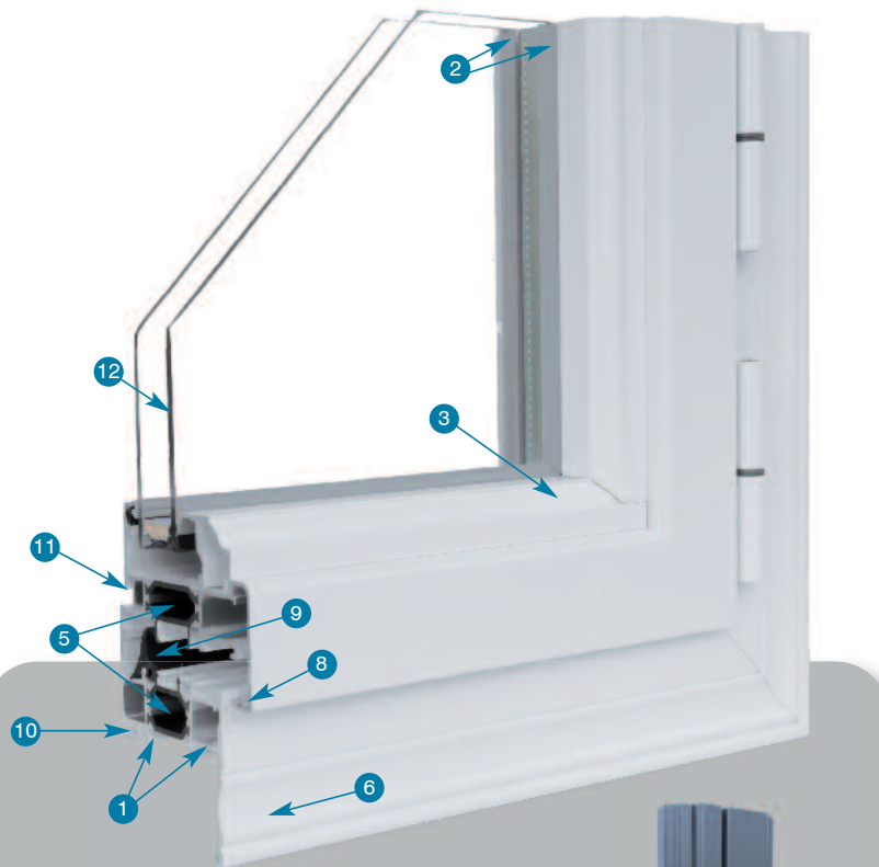
Montant central intérieur
