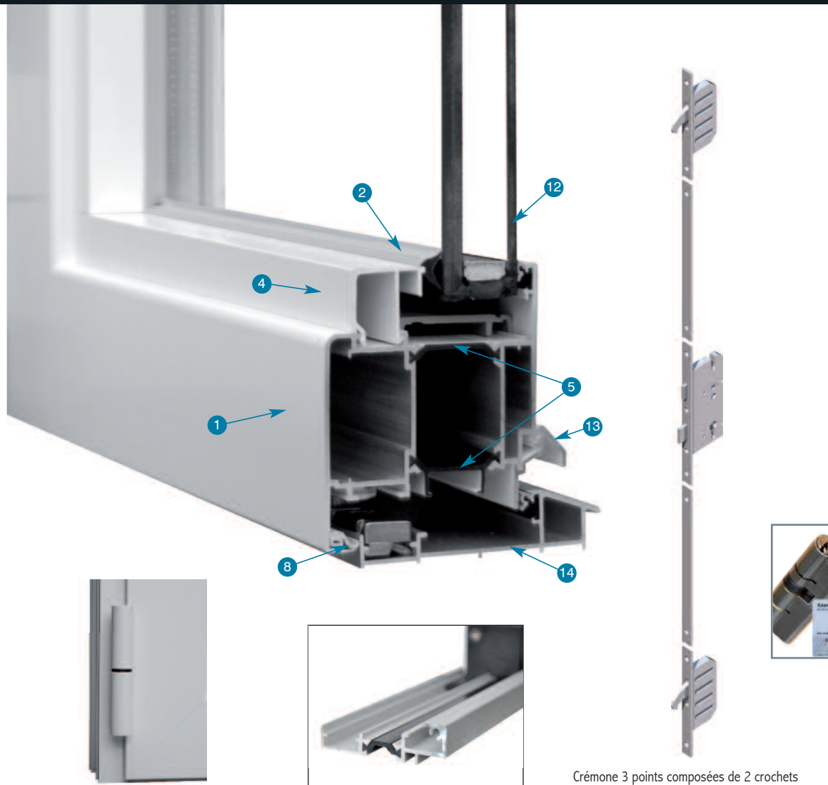
Le nouveau seuil à rupture de pont thermique
